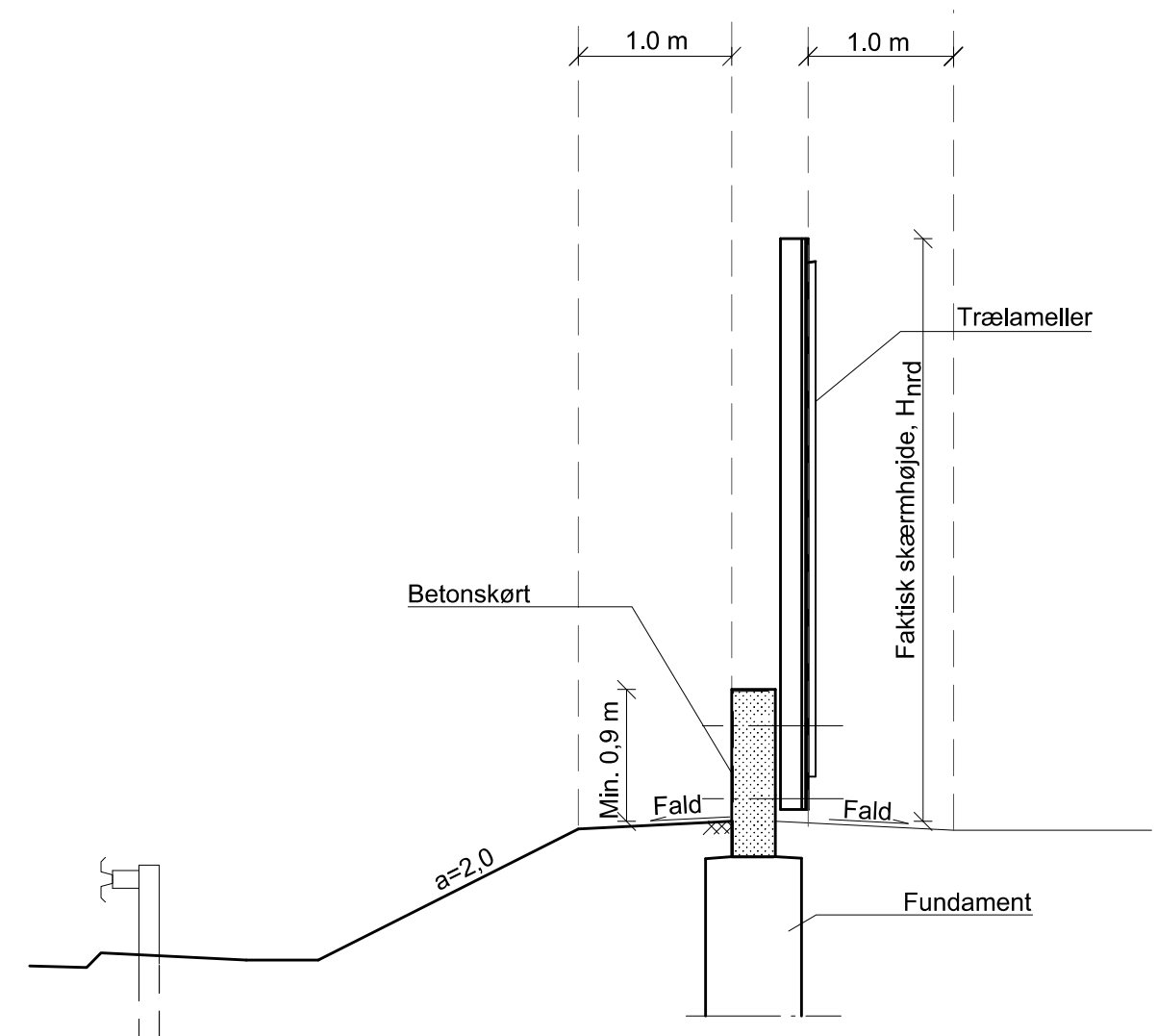
Tværsnit hvor vej ligger i afgraving, 1:50 Betonskørt mod vej
