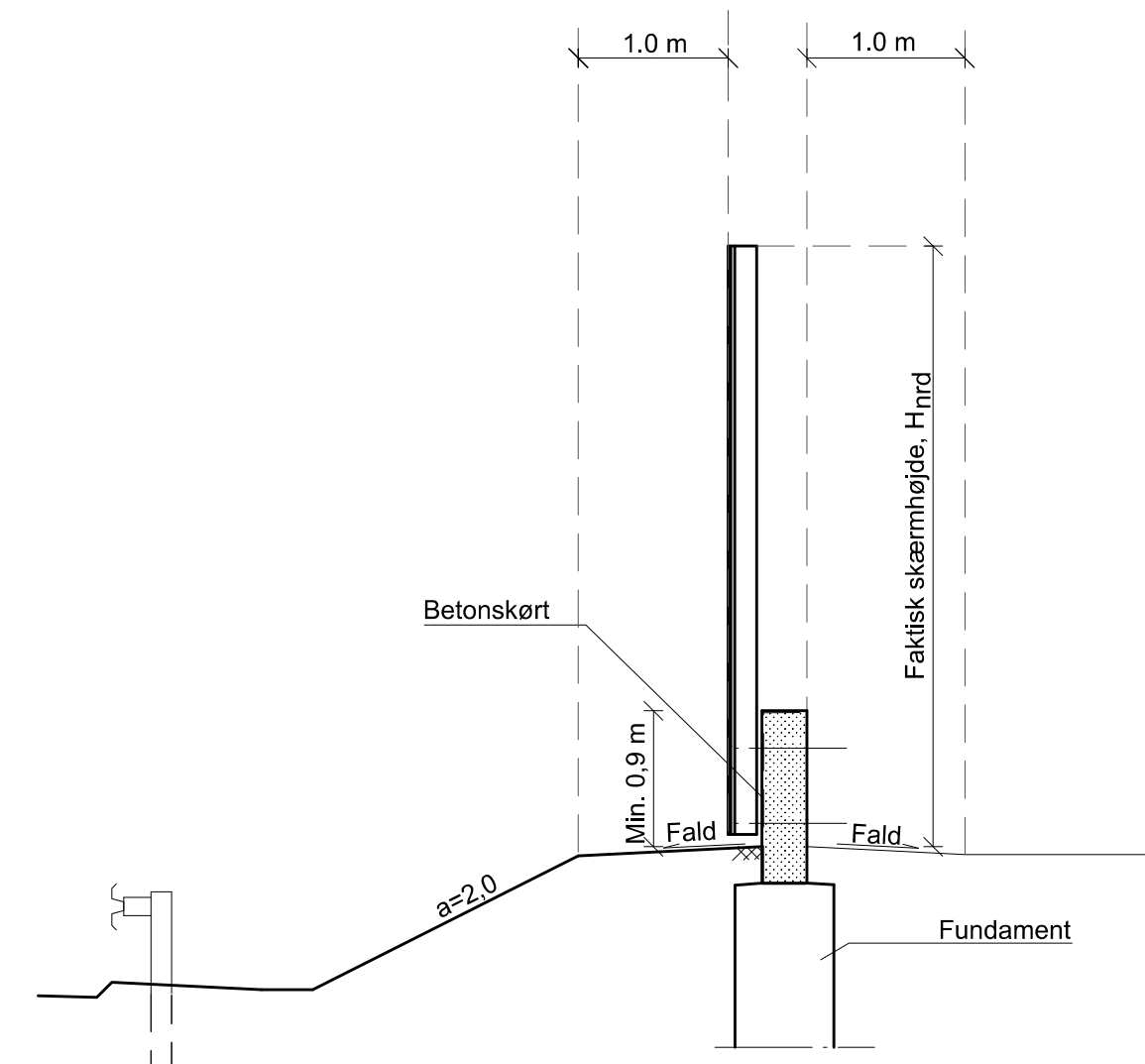
Tværsnit hvor vej ligger i afgravning, 1:50 Betonskørt mod naboareal
