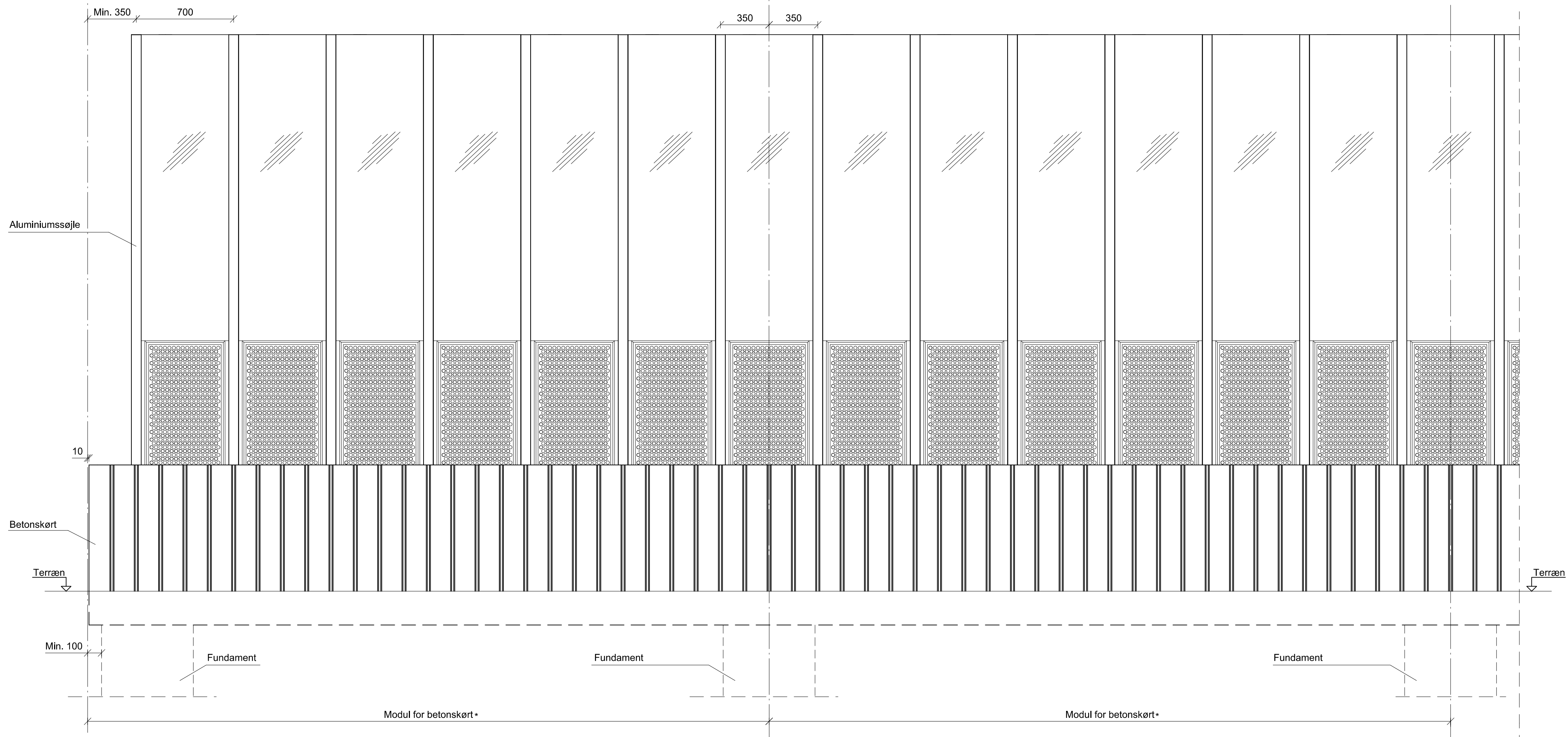
Opstalt ved ende af støjskærmsstrækning 1:20 Set fra vejside * Længden skal være delelig med 700 (f.eks. 3500 eller 4900)
