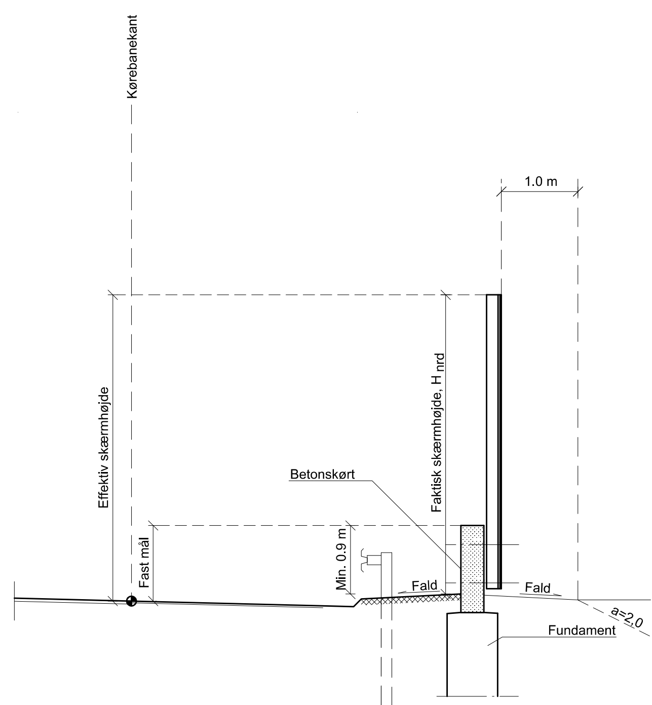
Tværsnit hvor vej er i terræn eller ligger på dæmning, 1:50
