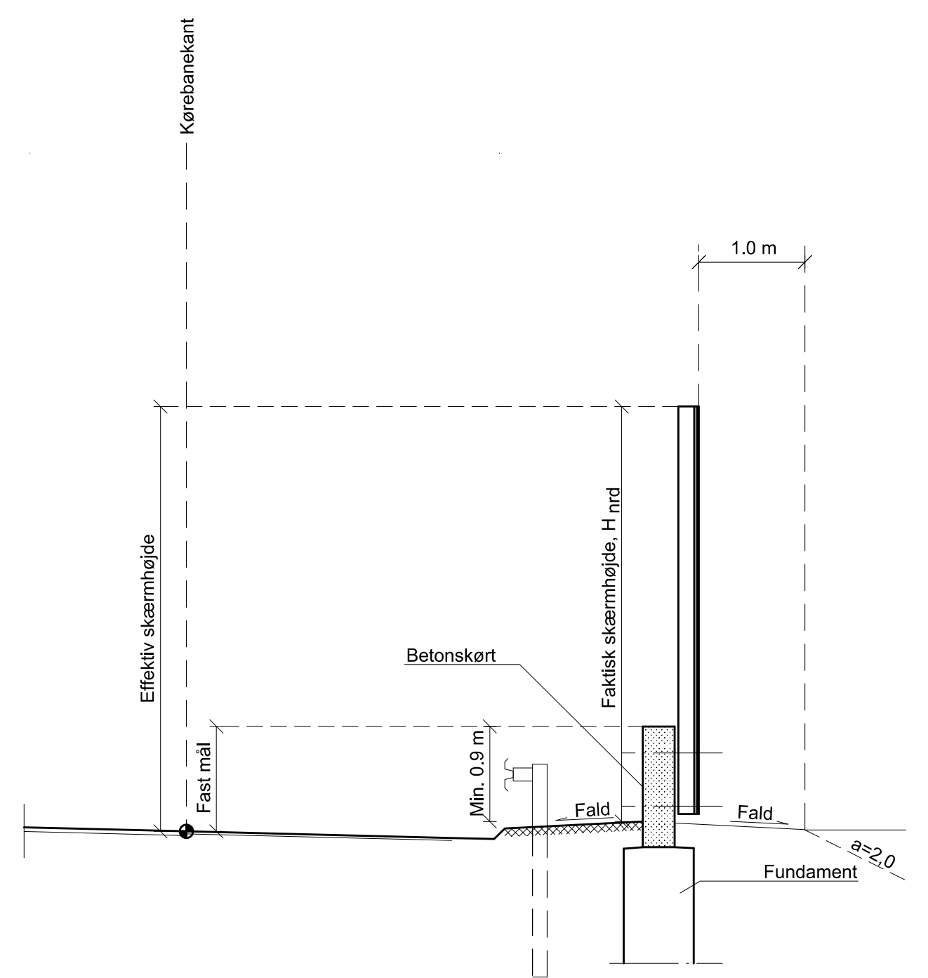
Tværnsnit hvor vej er i terræn eller ligger på dæmning, 1:50
