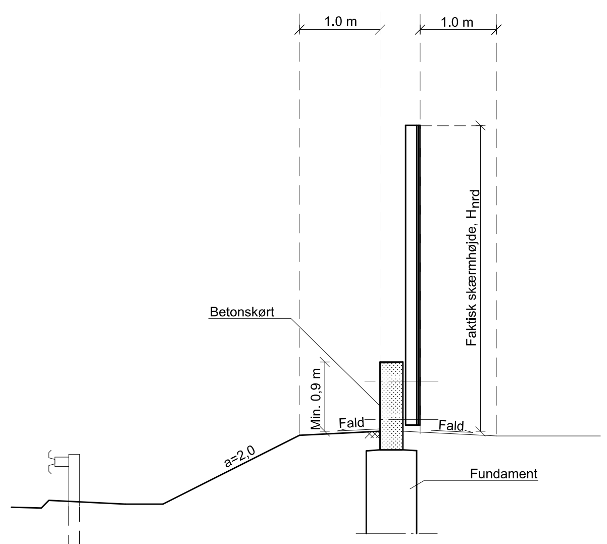
Tværnsnit hvor vej ligger i afgravning, 1:50 Betonskørt mod vej
