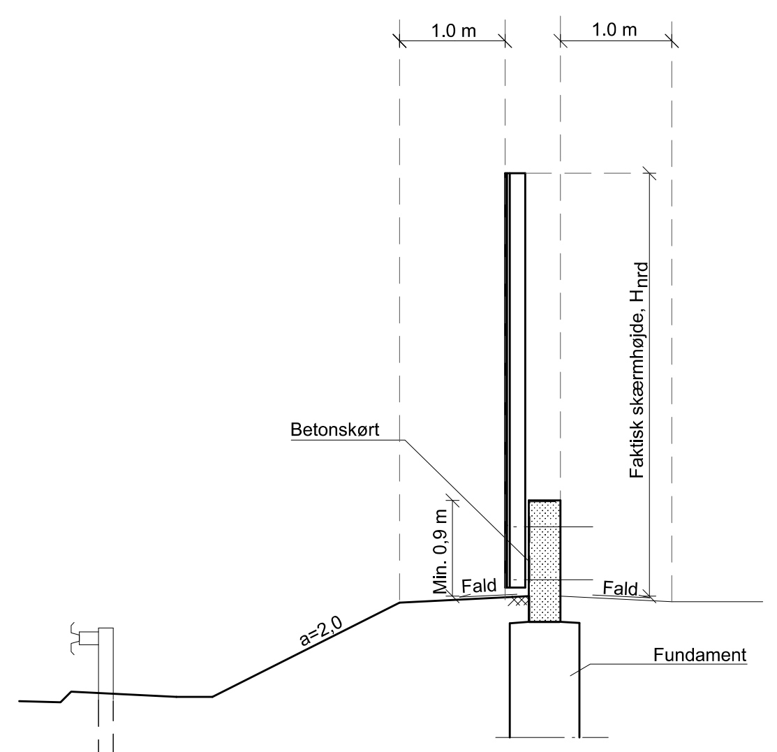
Tværnsnit hvor vej ligger i afgravning, 1:50 Betonskørt mod naboareal
