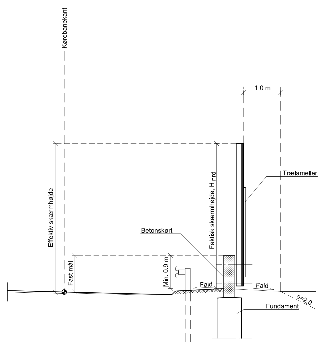
Tværsnit hvor vej er i terræn eller ligger på dæmning, 1:50
