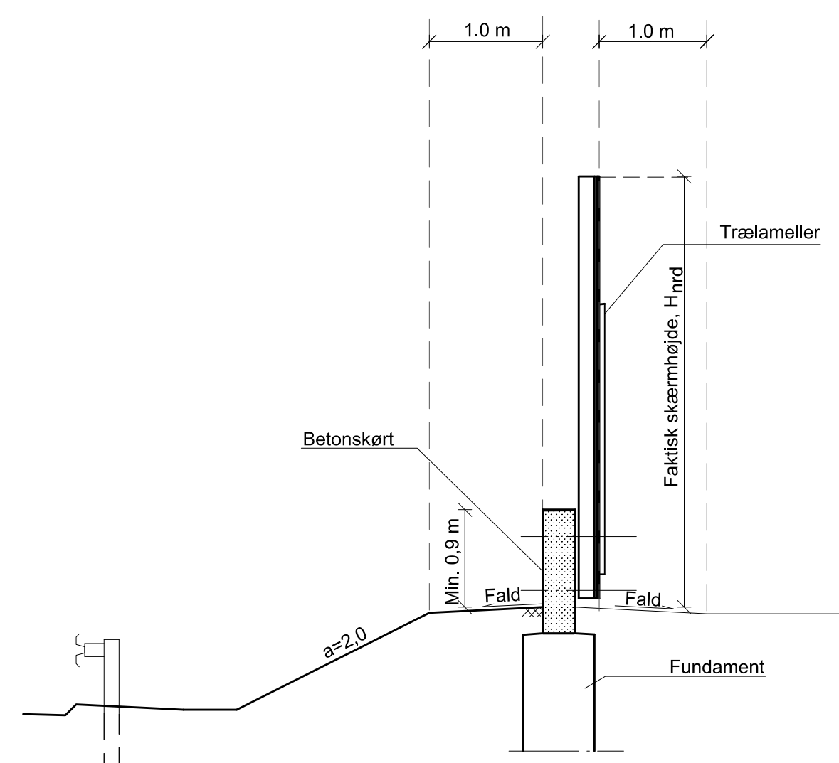
Tværsnit hvor vej ligger i afgravning, 1:50 Betonskørt mod vej
