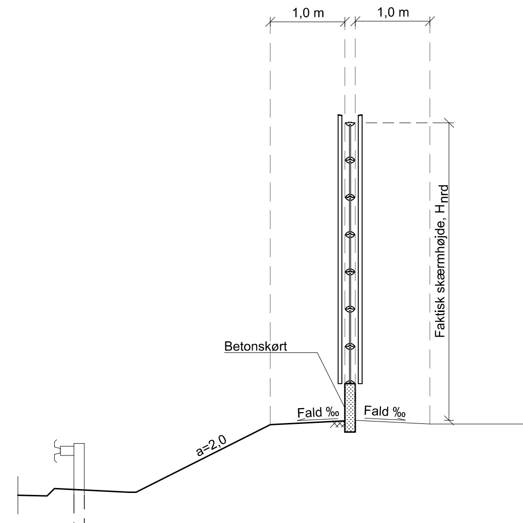
Tværsnit hvor vej ligger i afgraving, 1:50
