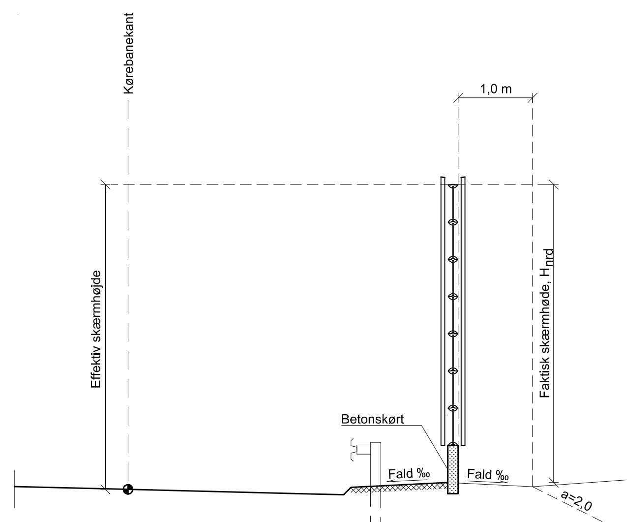
Tværsnit hvor vej er i terræn eller ligger på dæmning, 1:50
