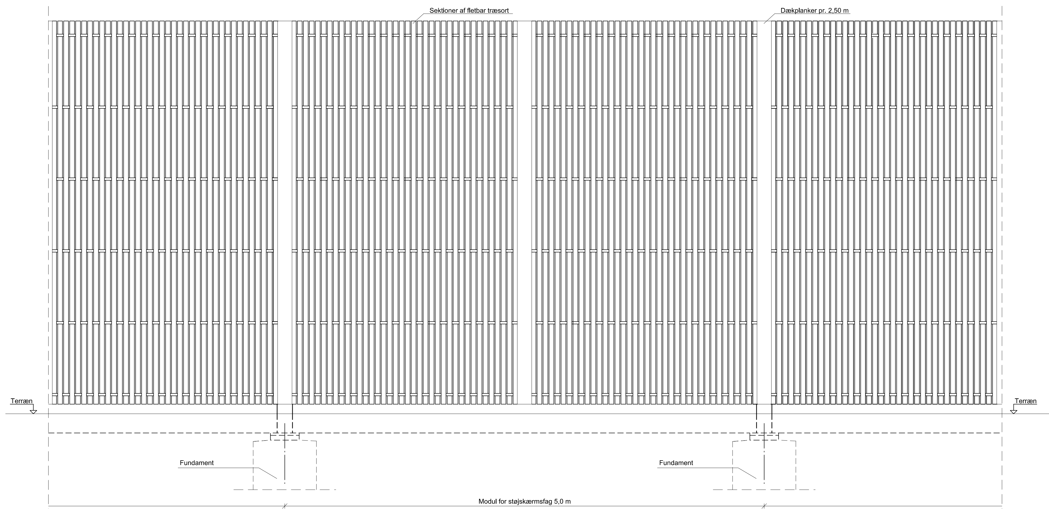
Opstalt af støjskærmsstrækning 1:20 Set fra vendside
