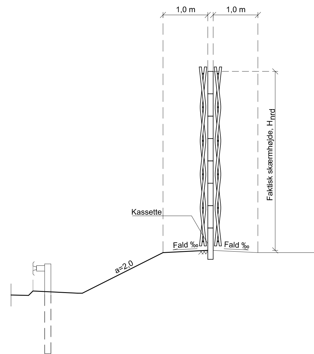
Tværsnit hvor vej ligger i afgravning, 1:50
