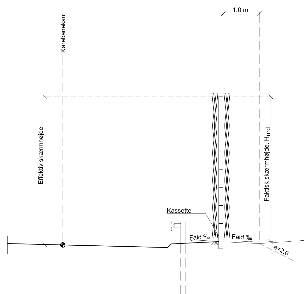
Tværsnit hvor vej er i terræn eller ligger på dæmning, 1:50
