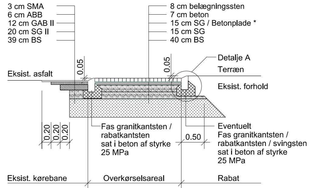
Tværsnit A - A Overkørselsareal
